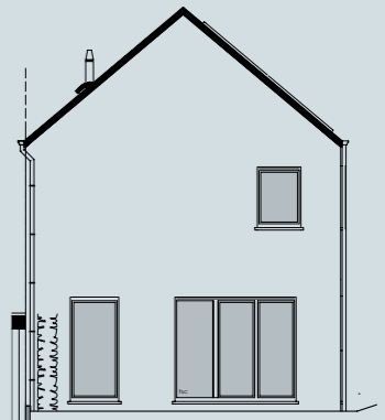
Façade arrière
