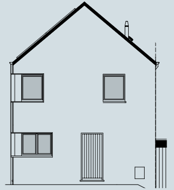
Façade avant
